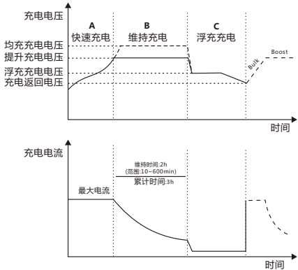
图1-5 铅酸电池充电阶段示意图
