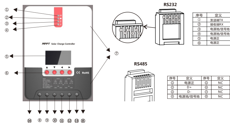
图1-1 控制器外观与接口
