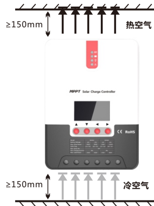
图2.1 安装和散热
