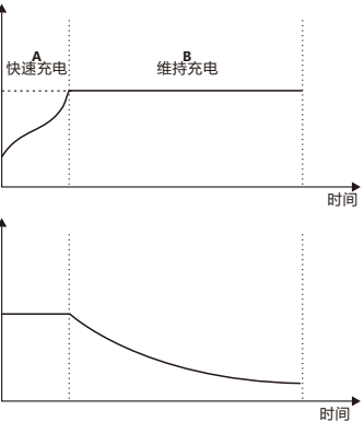
图1-6 锂电池充电阶段示意图
